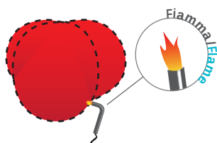
Applicazione di una fiamma ponendo il bruciatore a 45° Application of a flame by placing the burner to 45°
